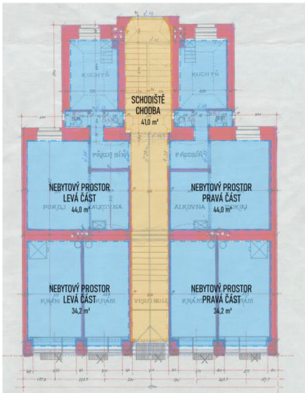
PŮDORYS 1.NP
