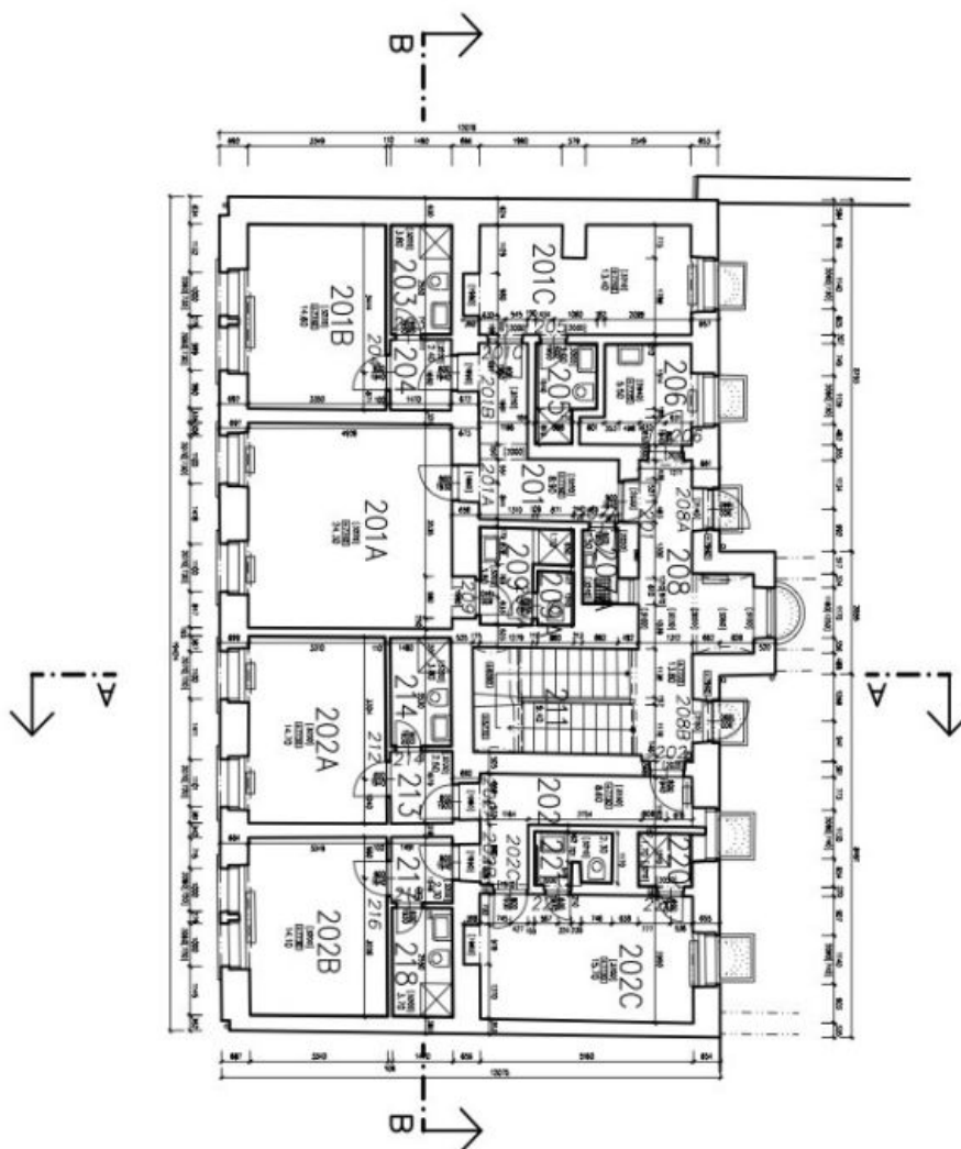
OBJEKT PENSION Hlinky 28a – půdorys II.patra 1:100
