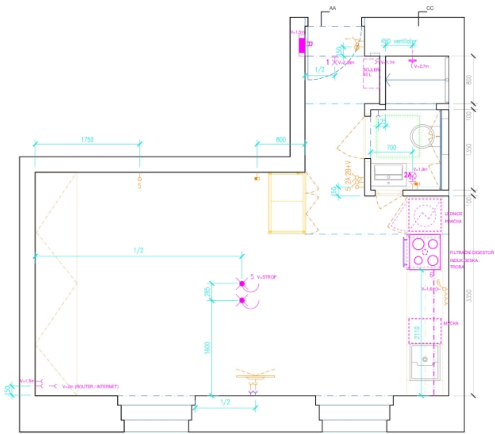
PŮDORYS BYTU
