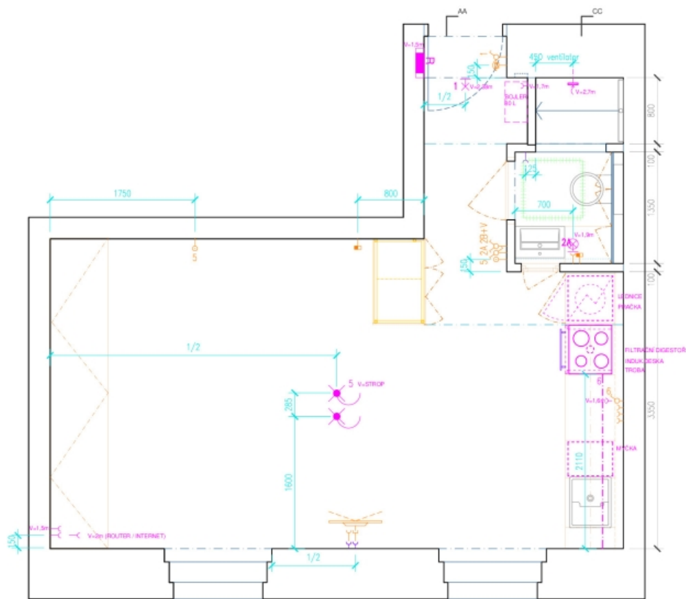
PŮDORYS BYTU
