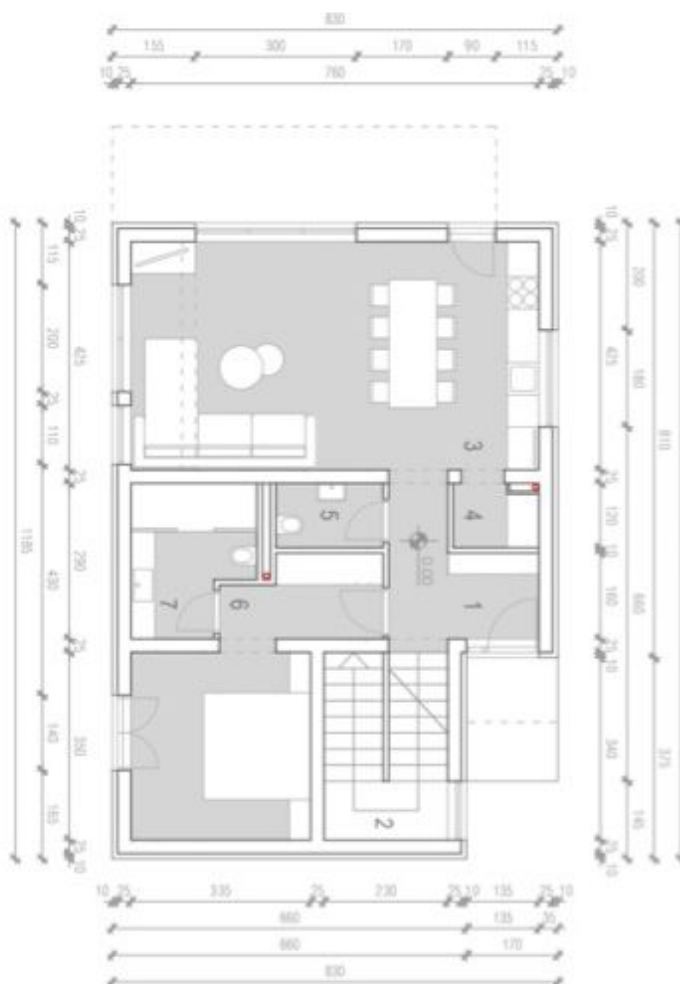
TLOCRT PRIZEMLJA
